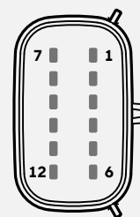
Molex MX150 12 ピン (背面)
